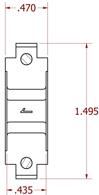
SECTION A-A SCALE 2 : 1
